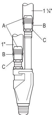
Fig. 3 Ejector cu conexiune din tub plastic
