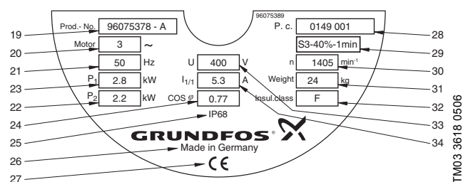
Фиг. 4 Табела с данни, двигател
