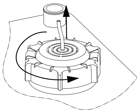
Фиг. 35 Отстраняване на сензора за ниво
