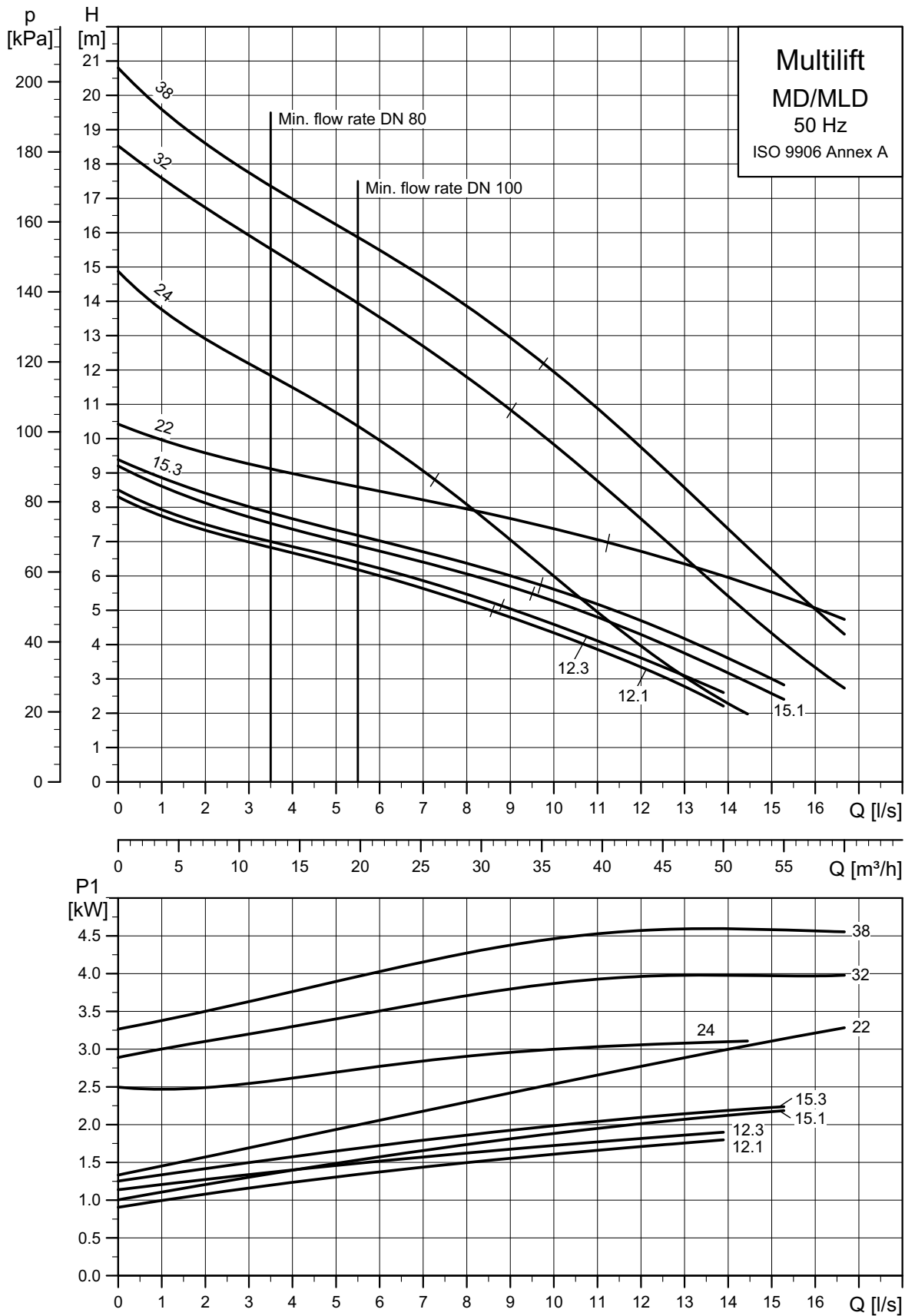
Фиг. 36 Работни криви
