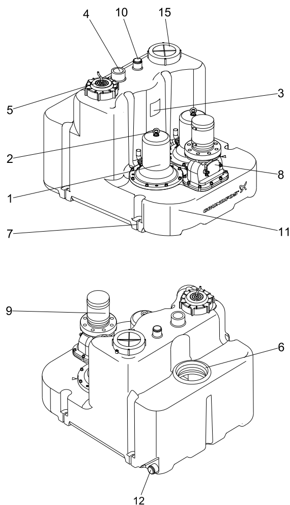
Фиг. 2 Multilift MLD, изглед отпред и отзад
