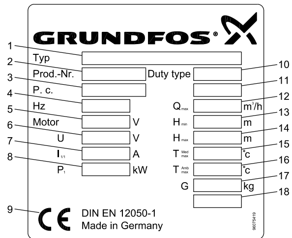
Фиг. 3 Табела с данни, подемна станция
