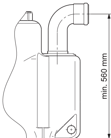
Фиг. 23 Минимално ниво на входа за MLD
