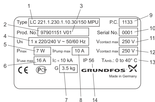
Фиг. 8 Пример за табела с данни на LC 221
