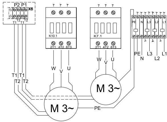
Фиг. 29 Диаграма на свързване, трифазно, Multilift MD/MLD.22.3.4 с контактори
