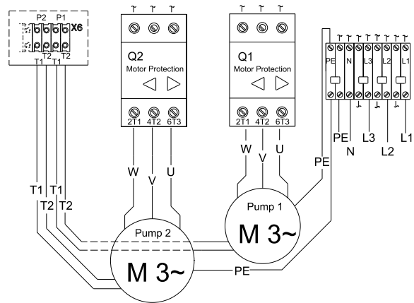
Фиг. 30 Диаграма на свързване, трифазно, Multilift MD/MLD.24.3.2, MD/MLD.32.3.2 и MD/MLD.38.3.2 с прекъсвач за защита на двигателя
