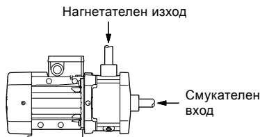
Фиг. 3 Смукателен вход и нагнетателен изход
