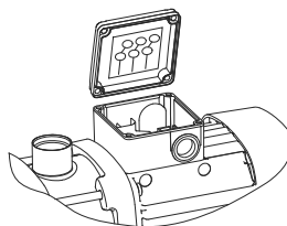
Фиг. 9 Схема на свързване
