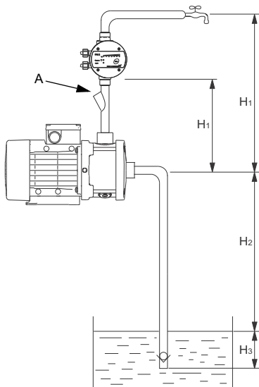
Фиг. 4 Препоръчителни тръбопроводи за самозасмукваща помпа
