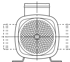
Фиг. 6 Позиции на клемната кутия
