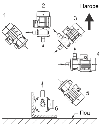
Фиг. 1 Положения на помпата
