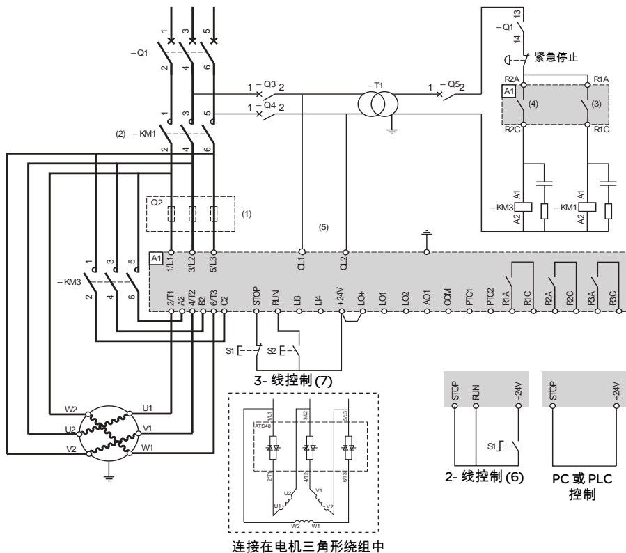
连接在电机三角形绕组中
